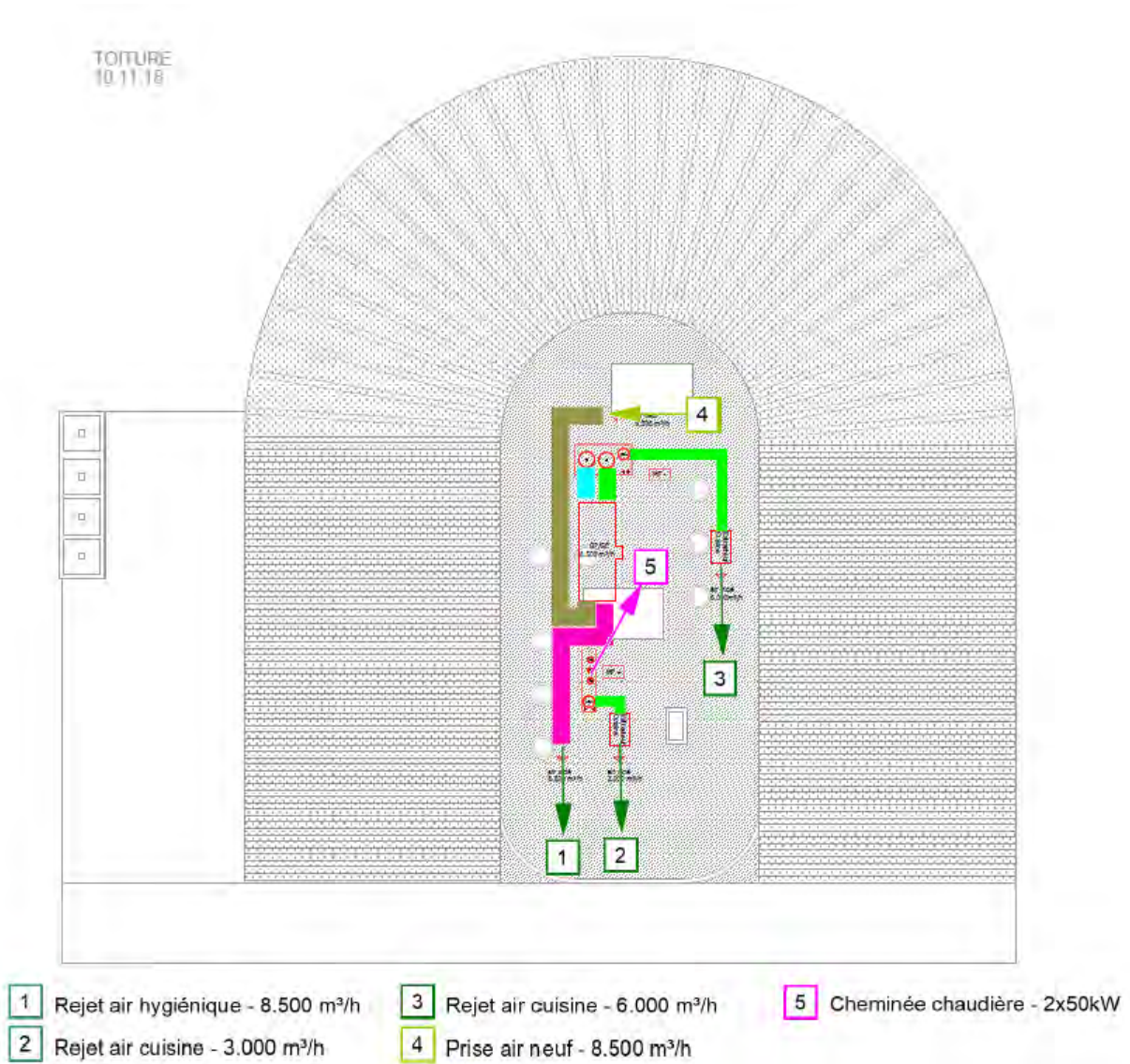
Figure 207: Localisation des prises d'air neuf au niveau de la façade et des rejets d'air au niveau de la toiture du restaurant (MK Engineering, 2018)
