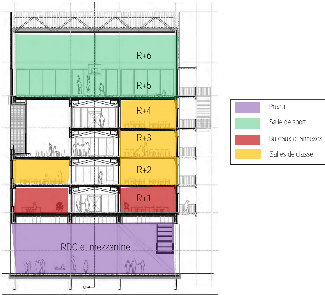
Figure 18 : Coupe de l'école D2-D3 et gabarits prévus (ARIES sur fond MSA, 2018)
