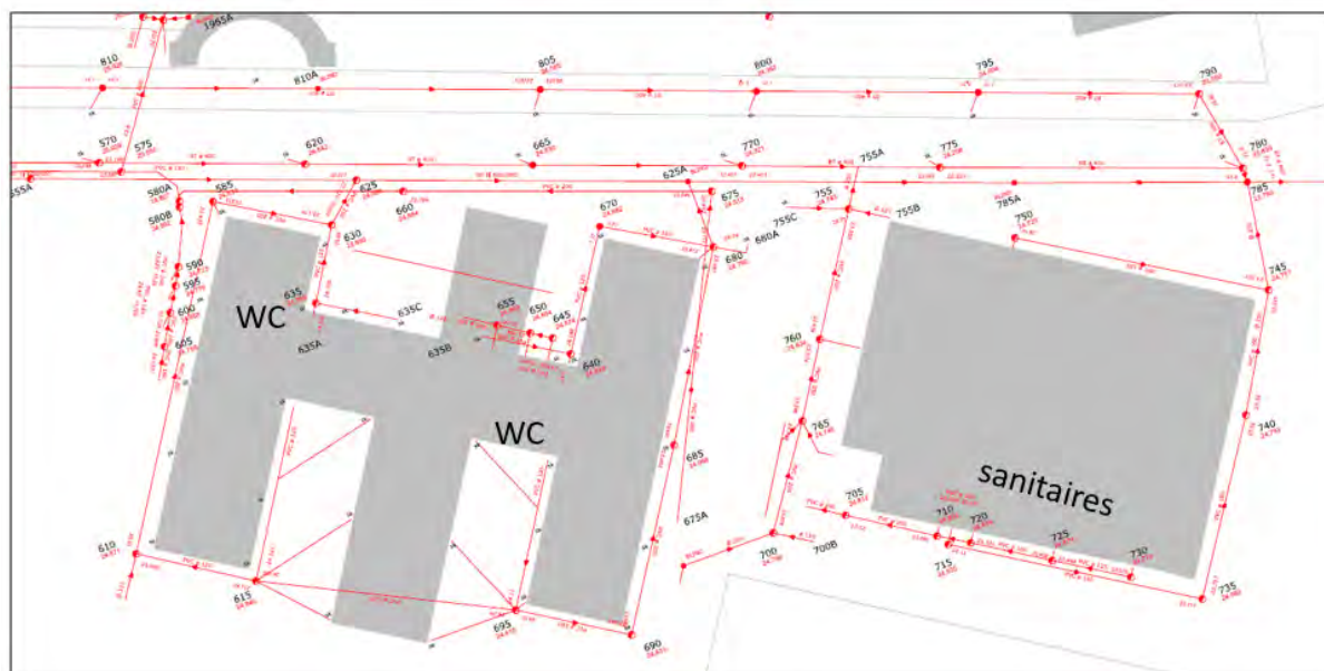
Figure 183 : Réseau d'égouttage existant actuellement dans le Sentier de la Drève (extrait de plan reçu de la part de WK Engineering, 2018)
