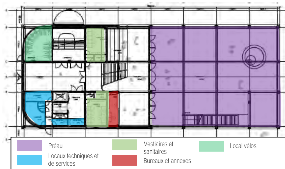
Figure 16 : Description de l'organisation spatiale intérieure du RDC (ARIES sur fond MSA, 2018)
