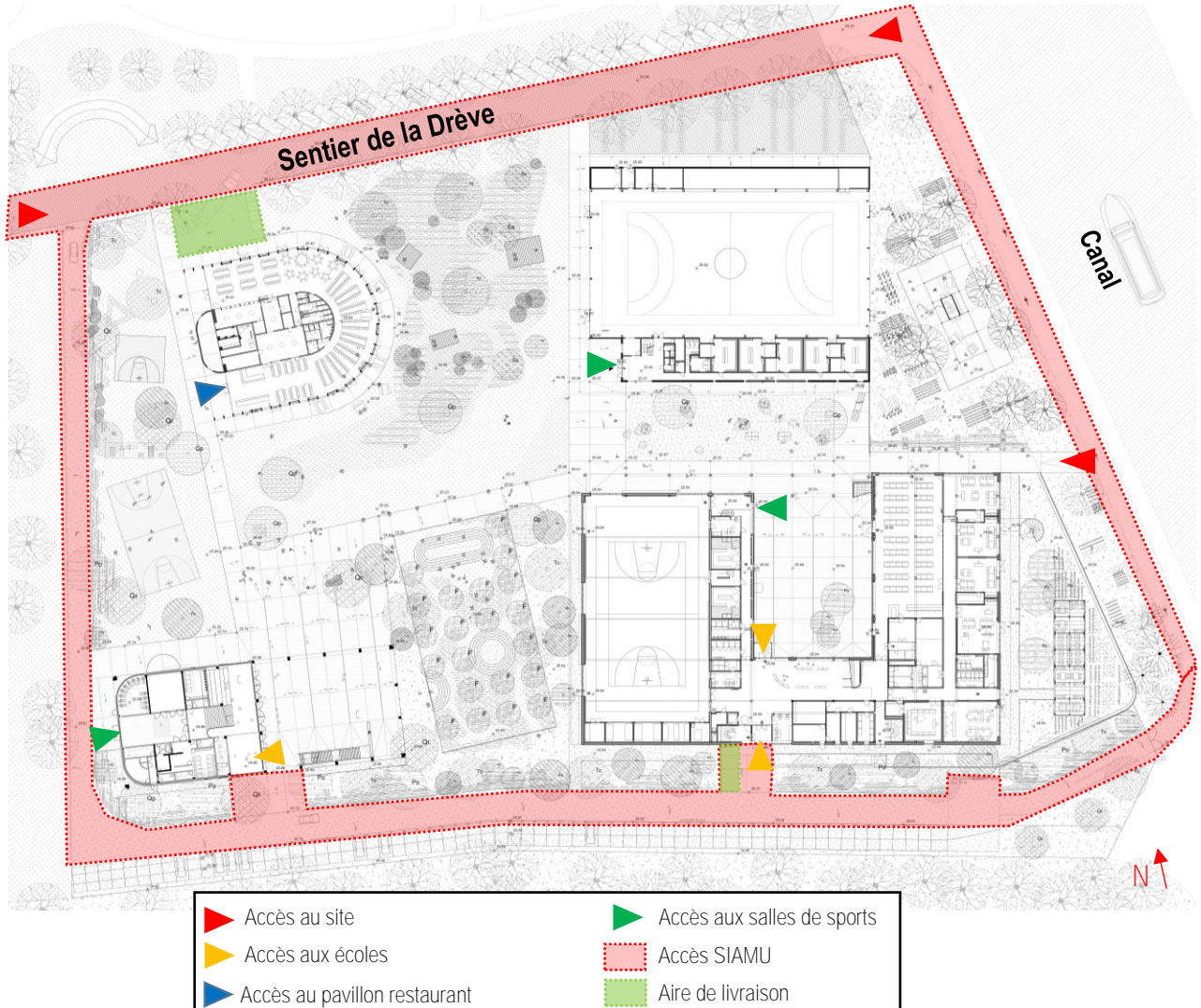
Figure 11 : Accès et cheminement en fonction des usagers et des bâtiments (ARIES sur fond 51NE4, 2018)
