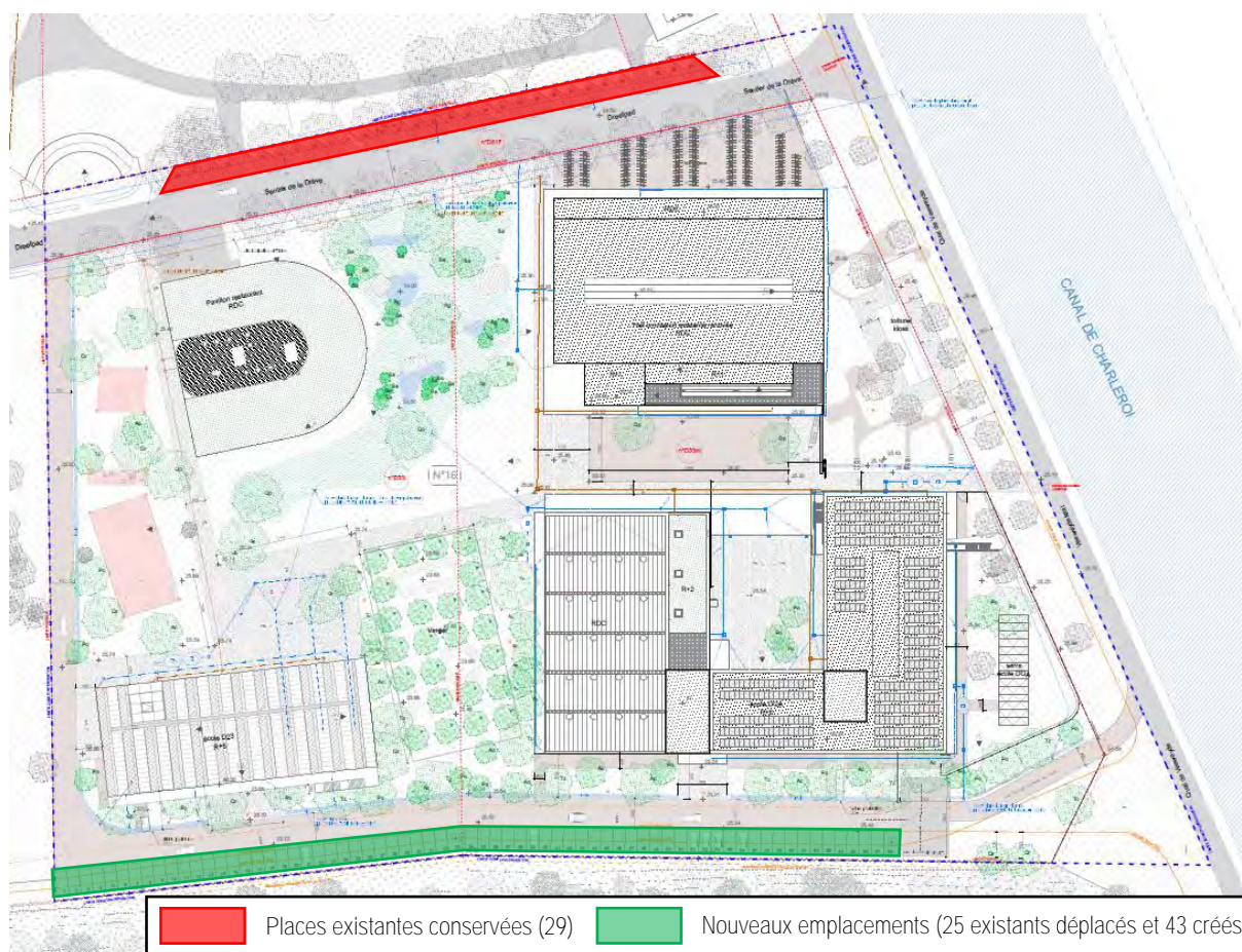
Figure 24 : Emplacements de parking en situation projetée (ARIES sur fond 51N4E, 2018)
