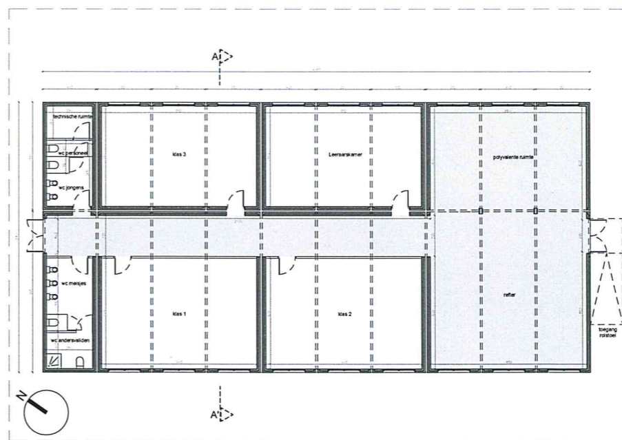
Grondplan 1:100e
